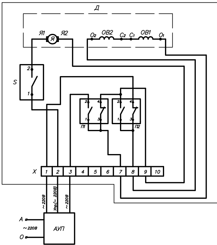
Схема электрическая принципиальная привода
